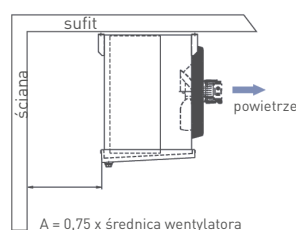
CHŁODNICA WYCIĄGOWA
