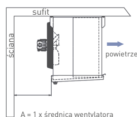
CHŁODNICA NADMUCHOWA
