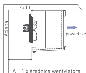
CHŁODNICA NADMUCHOWA
