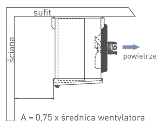
CHŁODNICA WCIĄGOWA
