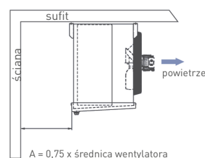
CHŁODNICA WYCIĄGOWA
